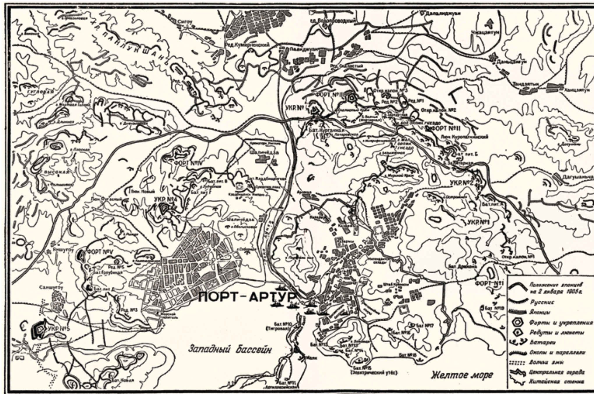
Карта фортификационных сооружений оборонительной линии Порт-Артура
